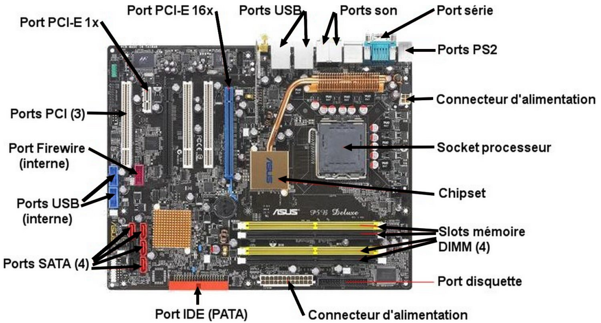
FIGURE 71 – Connectivité interne et externe d'une carte mère
