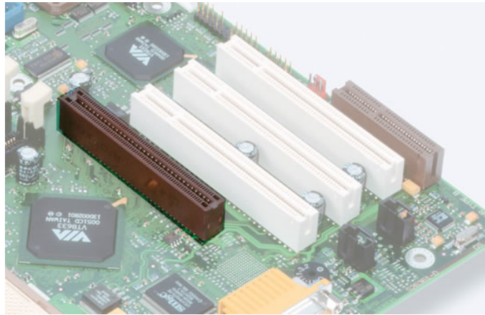
FIGURE 67 – Connecteur AGP
