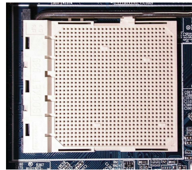
FIGURE 63 – Socket 939 pour processeur AMD
