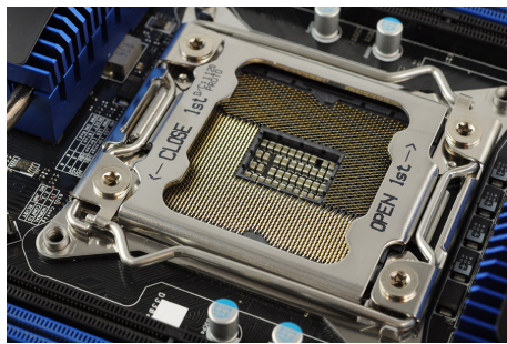
FIGURE 62 – Socket LGA2011 pour processeur Intel
