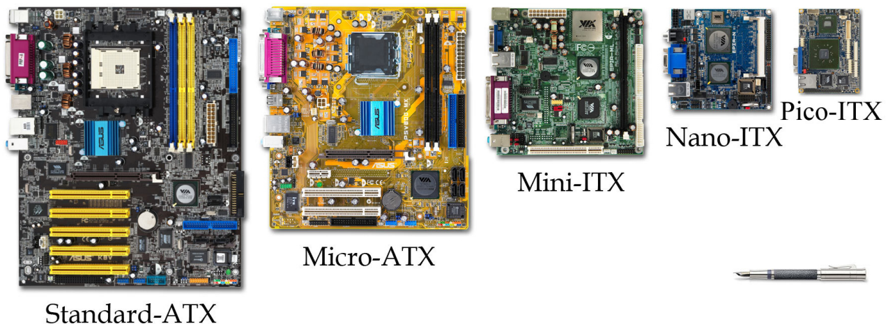
FIGURE 41 – Quelques carte-mères de « facteurs de forme » différents
