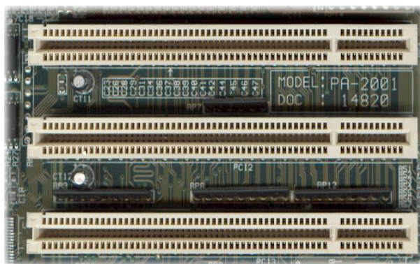
FIGURE 66 – Connecteurs PCI
