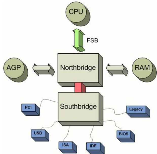
FIGURE 61 – Rôle du Northbridge et Southbridge
