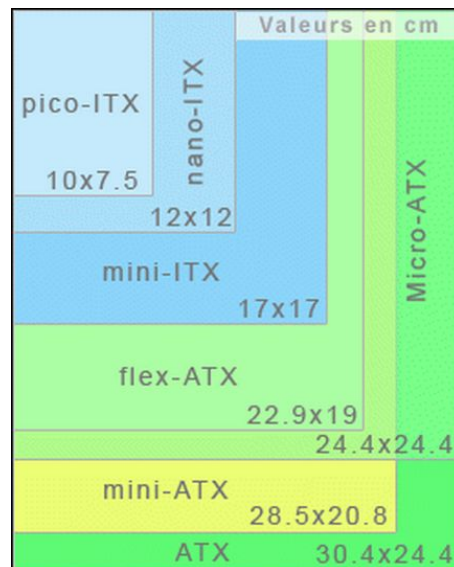
FIGURE 59 – Les différents facteurs de forme
