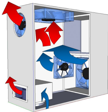
FIGURE 45 – Aération dans un PC
