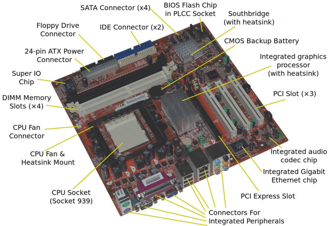
FIGURE 72 – Carte-mère Acer E360 Socket 939
