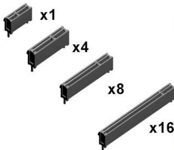
FIGURE 68 – Connecteurs PCI-Express
