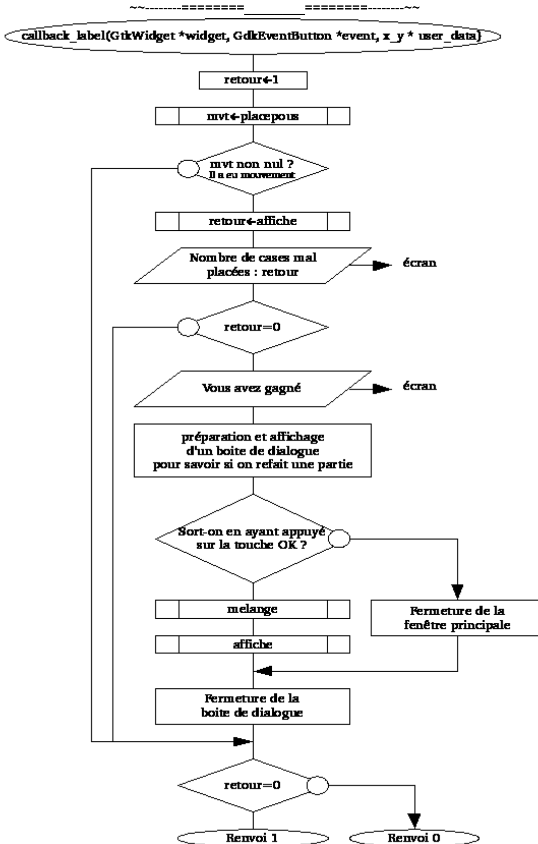
La fonction callback_label qui renvoie 1 si le taquin est fini, 0 sinon.
