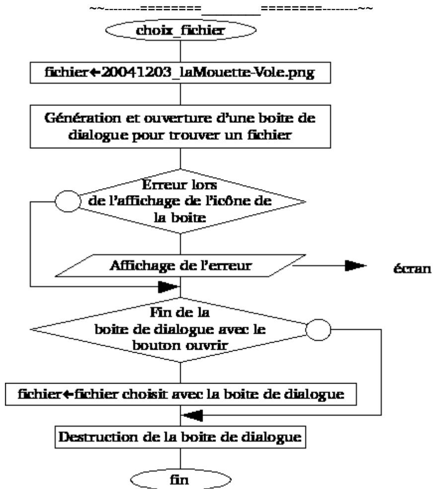
La fonction choix_fichier
