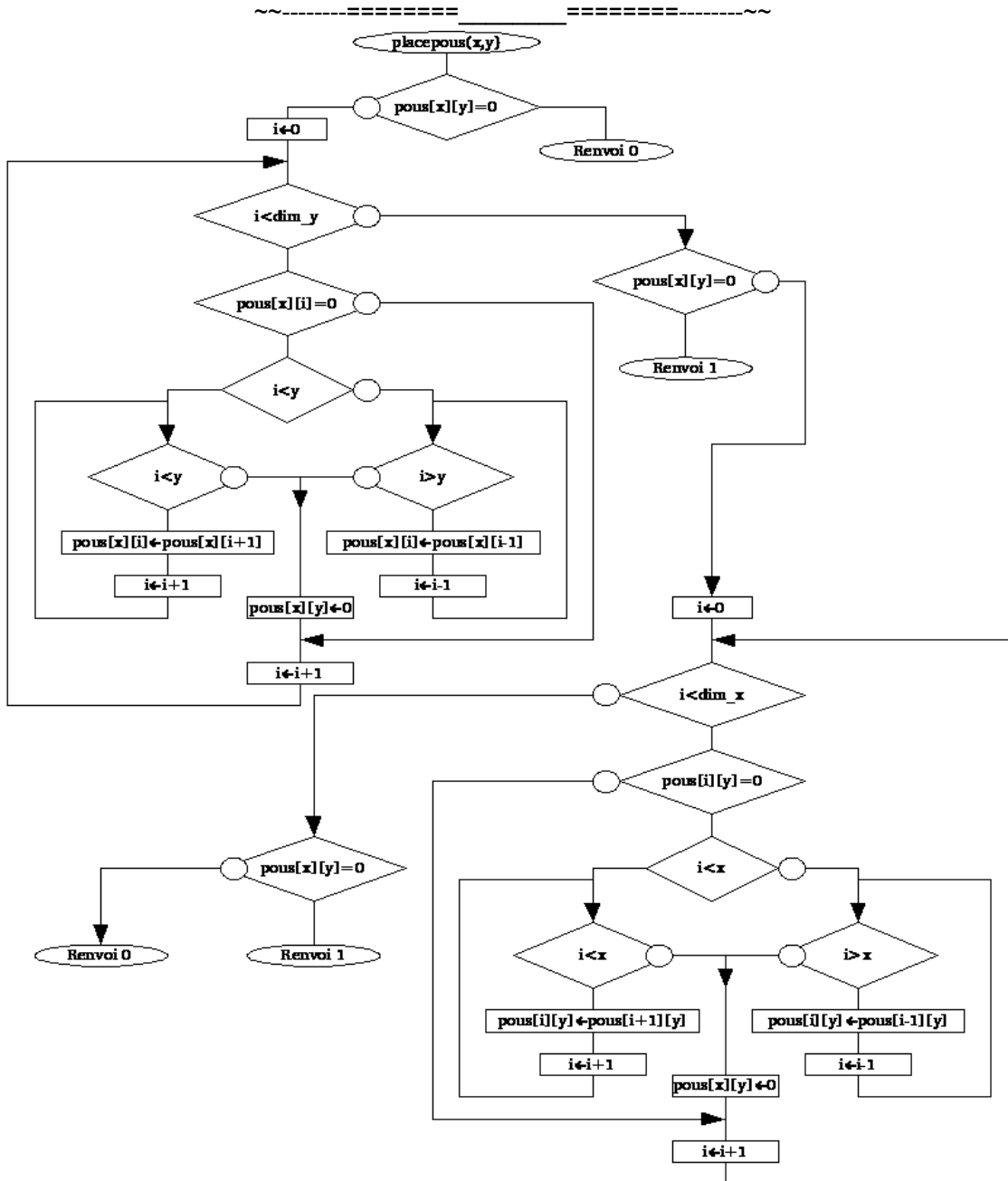
La fonction placepous qui renvoie 1 s'il y a eu un mouvement.
