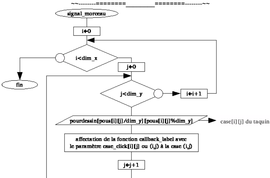
La fonction signal_morceaux
