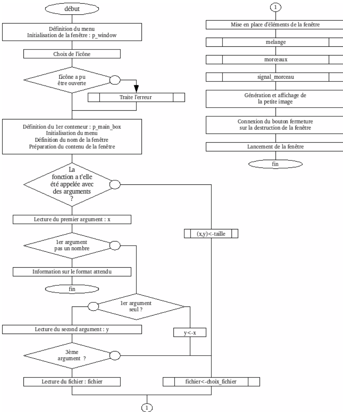
Le corps du programme
